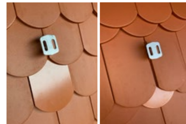
(Bild 3, links Doppeldeckung, rechts Kronendeckung)
