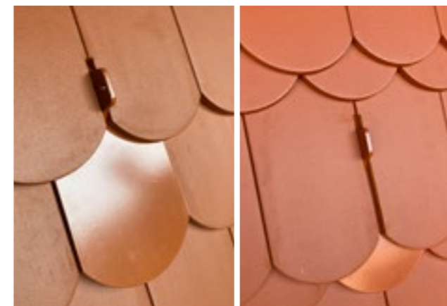
(Bild 2, links Doppeldeckung, rechts Kronendeckung)
